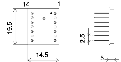
Корпус 151.15-8 вид со стороны выводов
